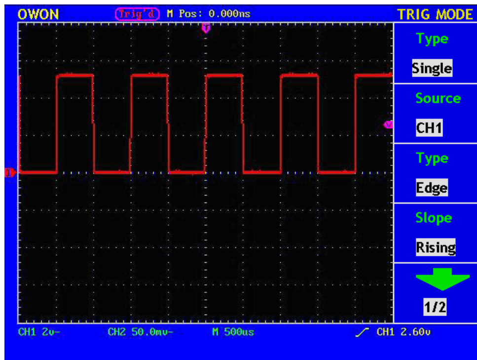
Fig.6 Auto set
